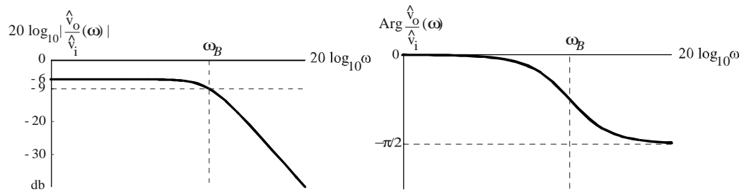
Figura 6.6: Módulo e argumento de \hat{v}_o / \hat{v}_i para o circuito da figura anterior
